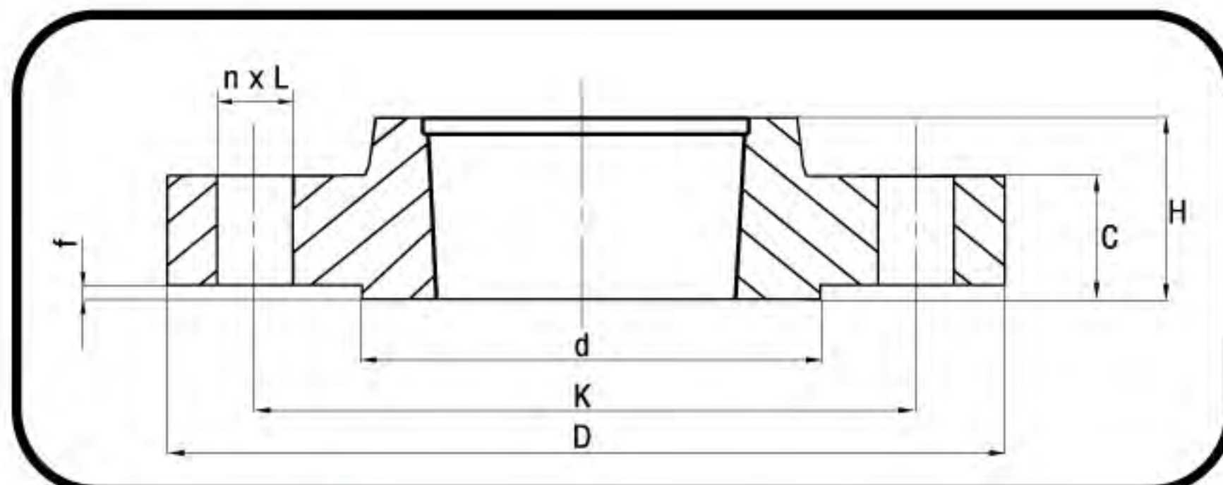
▲ Dimensions Cast Iron Flange มิติหน้าแปลนเหล็ก (mm.)
