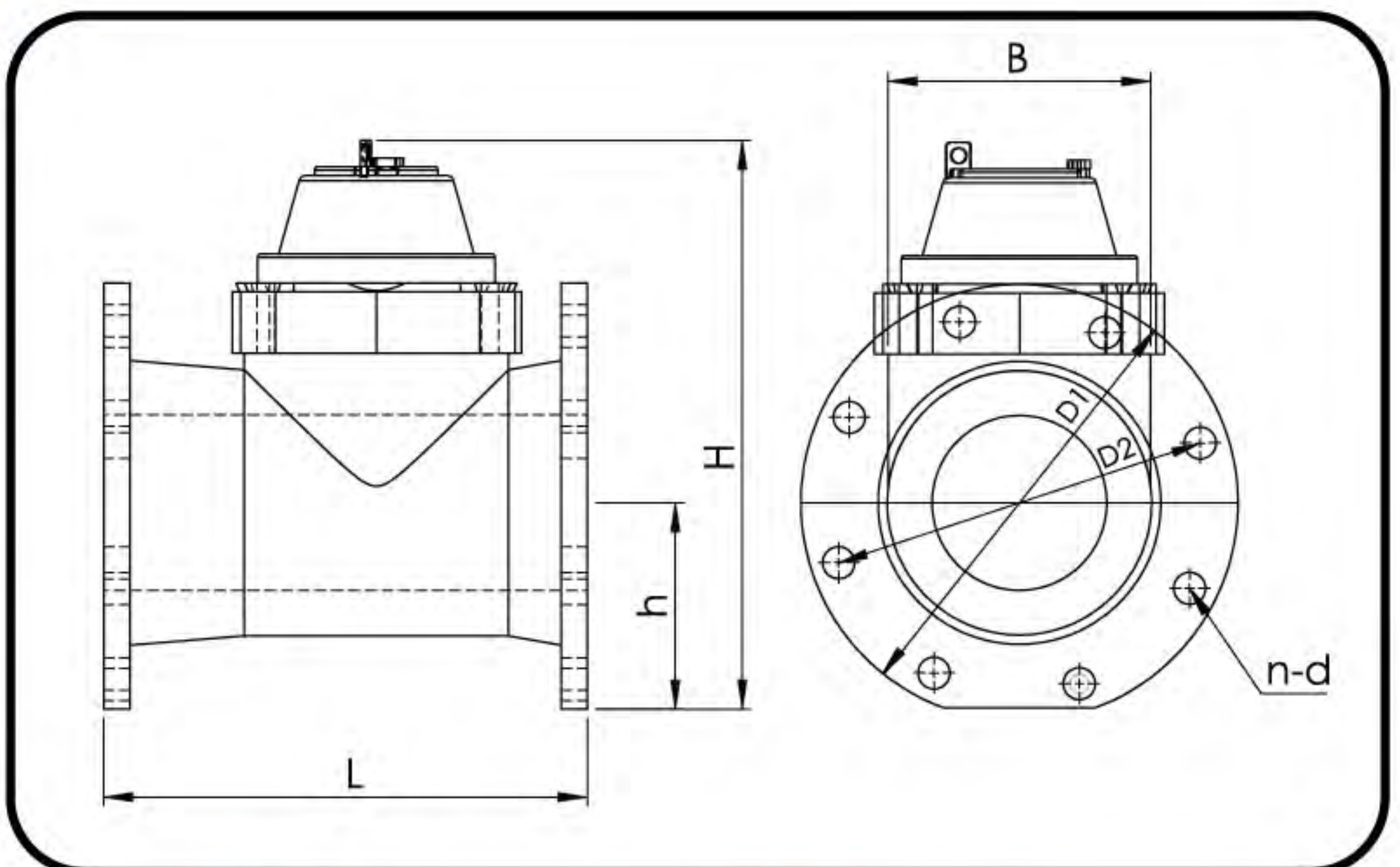
▲ Dimensions มิติ (mm.)
